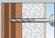
1 Bohrloch herstellen.
