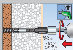
2 Putz auffräsen.
